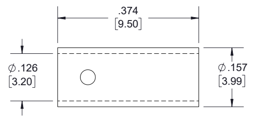
FERRULE
