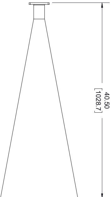
WR-430 STD CPRF FLANGE UG-1711/U
