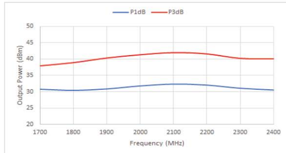
P1dB & P3dB
