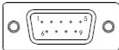
VIEW A-A
