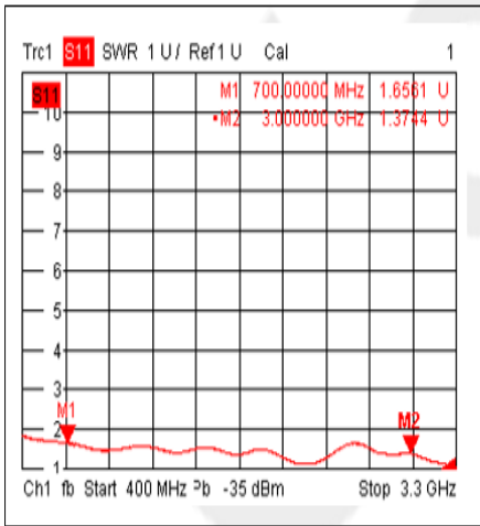
Input VSWR@-40°C
