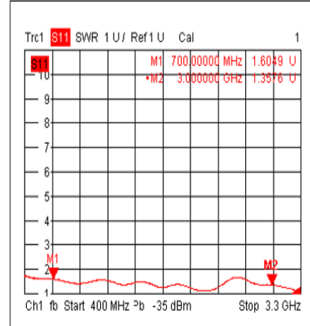
Input VSWR@+70°C
