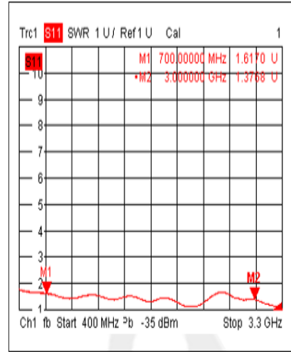
Input VSWR@+25°C
