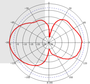
V-Plane: 928MHz
