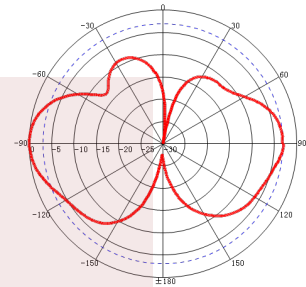
V-Plane: 902MHz
