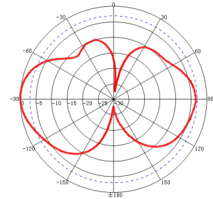
V-Plane: 915MHz
